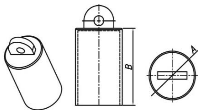
钢丝管护套 (材质: PVC)
